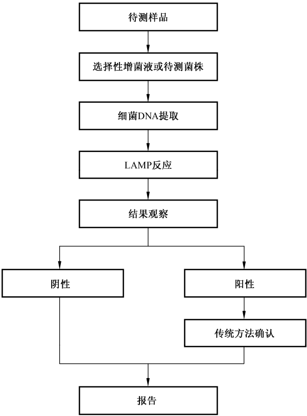
图 1 食品中空肠弯曲菌 LAMP 检测程序
